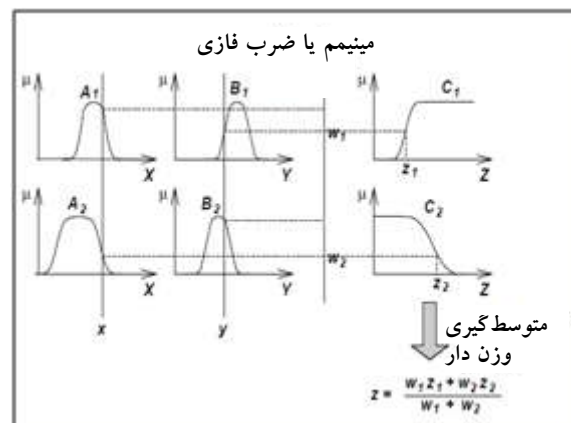
شکل ۲. مدل تسوکاموتو
