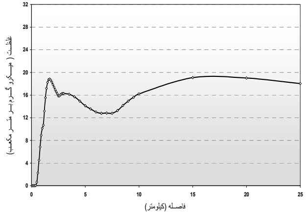
نحوه پراکنش NO_x نیروگاه رامین اهواز
