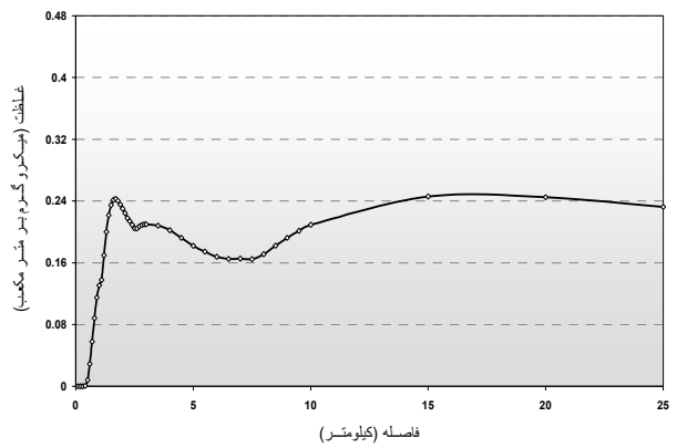
نحوه پراکنش SO_2 نیروگاه رامین اهواز
