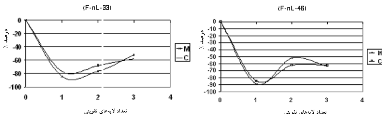
شکل ۷ درصد اختلاف انرژی جذب شده نمونه های تقویت شده نسبت به نمونه های شاهد
