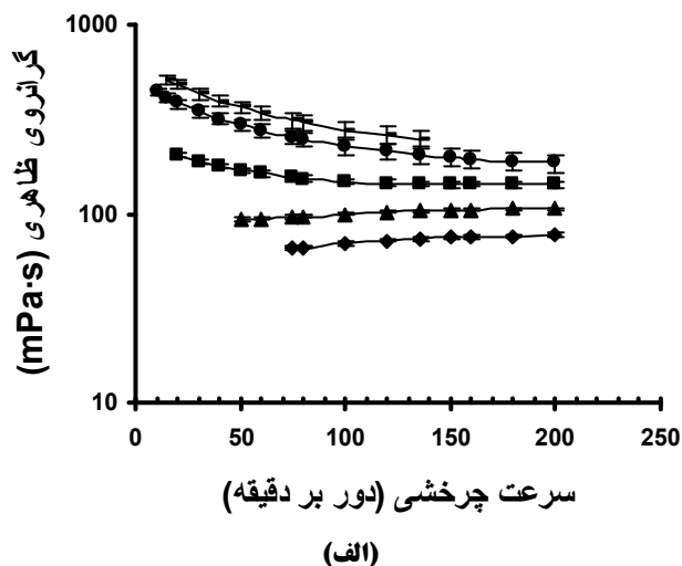
شکل ۲. نمایش رفتار جریان محلول‌های پودر ثعلب در غلظت‌های مختلف (۶، ۵، ۴، ۳، ۲، ۱ گرم در لیتر) در دمای ۲۵ درجه سانتی‌گراد و پ هاش ۷ (الف) سرعت چرخشی در مقابل گرانیوی ظاهری (ب) سرعت برشی در مقابل گرانیوی ظاهری.
