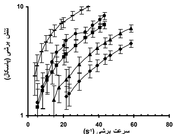
شکل ۳. نمایش تغییرات سرعت برشی در مقابل تنش برشی در محلول‌های پودر ثعلب در غلظت‌های مختلف (۶، ۵، ۴، ۳، ۲، ۱ گرم در لیتر) در دمای ۲۵ درجه سانتی‌گراد و پ هاش ۷.
