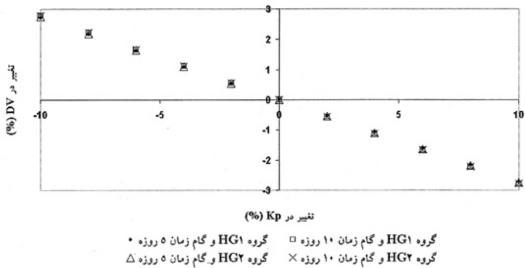
شکل ۳- آنالیز حساسیت معادله ۳- نسبت به تغییرات ضریب Kp
