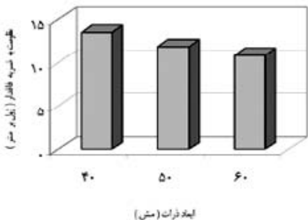
شکل ۴- اثر مستقل ابعاد ذرات آرد چوب بر مقاومت به ضربه فاقدار چند سازه آرد چوب / پلی پروپیلن
