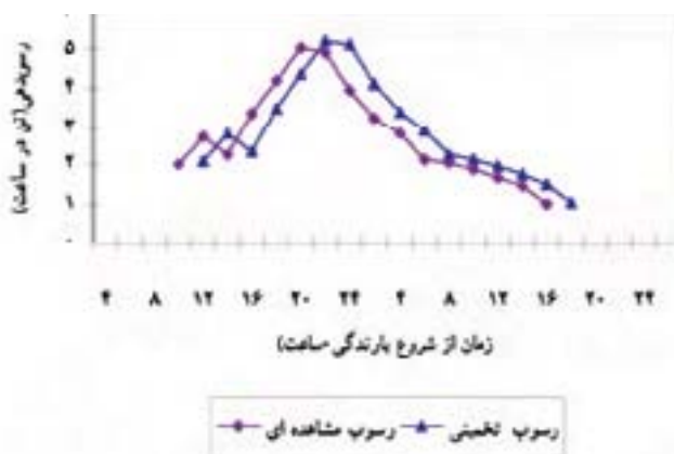
شکل ۴: منحنی‌های رسوب مشاهده ای و تخمینی ناشی از برازش مدل رگرسیونی گسسته برای رویداد بارندگی ۸۲/۱۰/۱۷
