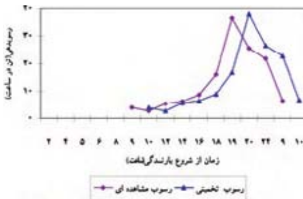
شکل ۷: منحنی‌های رسوب مشاهده‌ای و تخمینی
