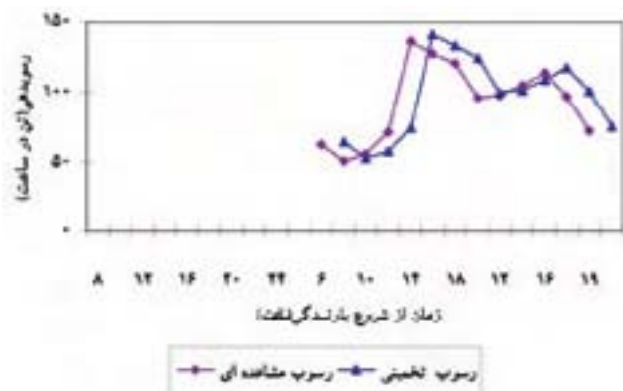
شکل ۸: منحنی‌های رسوب مشاهده‌ای و تخمینی
