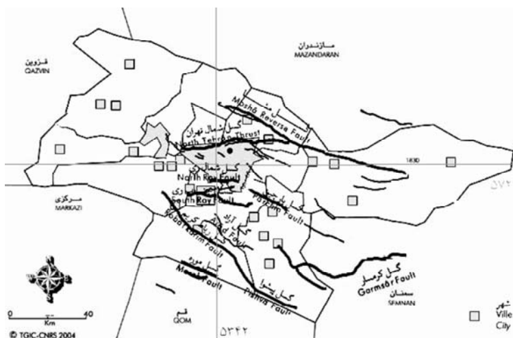
شکل ۱ نقشه پراکنش گسل‌ها نسبت به شهر تهران [۱۰]
