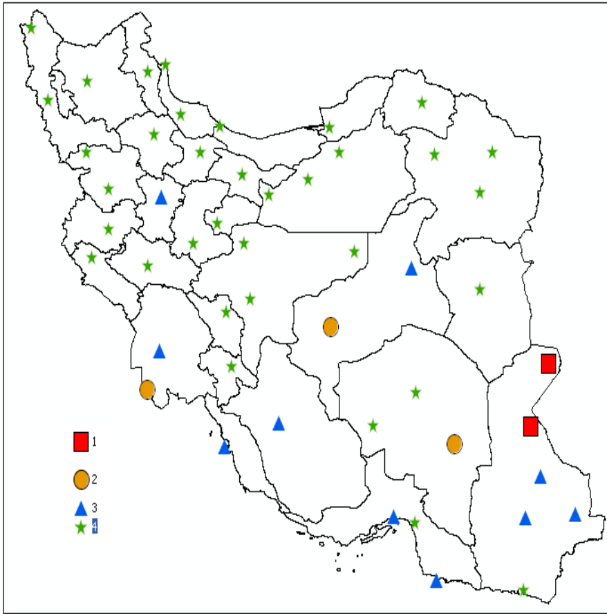
شکل ۴ نقشه پراکنده‌گی طبقه‌بندی ایستگاه‌های مطالعه‌شده بر اساس فراوانی ماهیانه طوفان‌های گرد و خاک معلق در هوا
