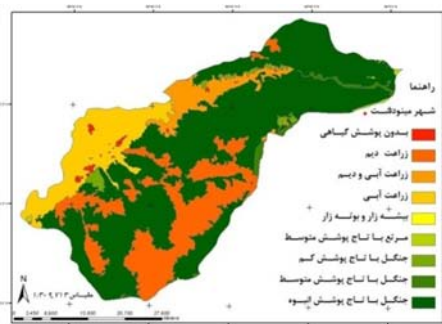
شکل 7 پوشش گیاهی
