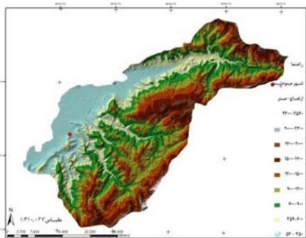
شکل 3 طبقات ارتفاعی
