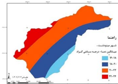
شکل 10 میانگین دما
