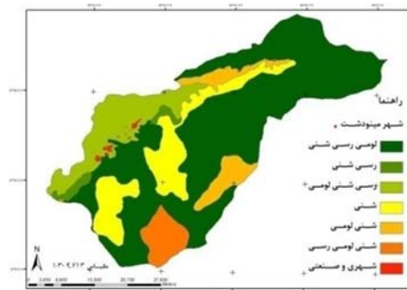
شکل 6 بافت خاک
