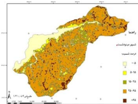
شکل 4 درصد شیب
