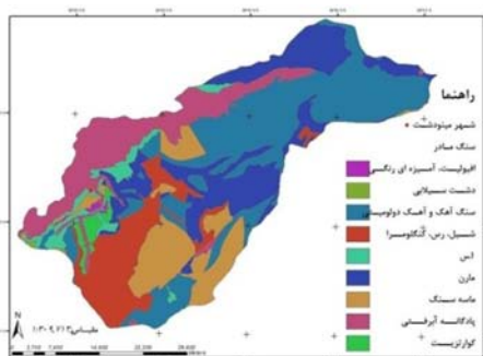
شکل 9 واحدهای سنگ‌شناسی
