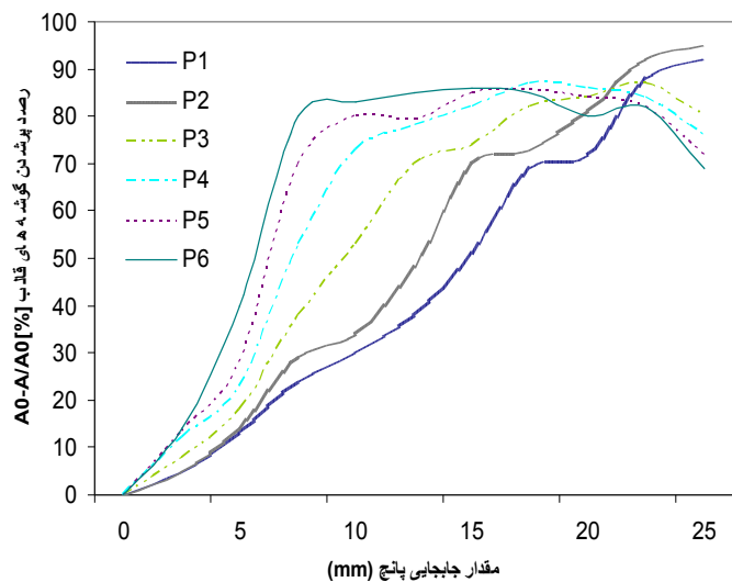
شکل ۱۲ درصد پر شدگی گوشه قالب برای تمامی مسیرهای فشار.
