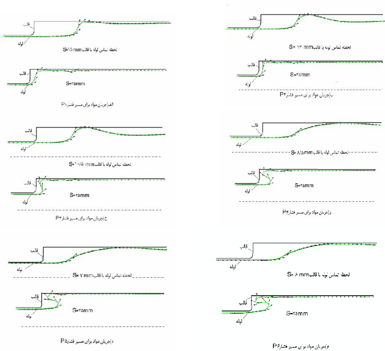
شکل ۹ بردارهای جریان مواد مربوط به ناحیه تغییر شکل لوله در لحظه تماس اولیه لوله و قالب و زمان پایان فرآیند، مقدار جابجایی سنه S .
