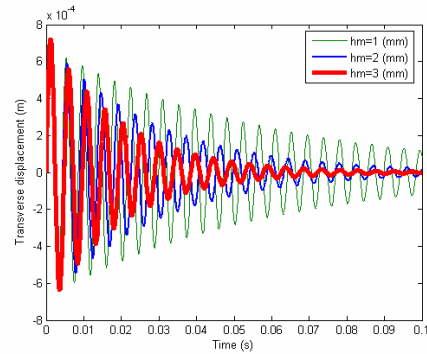
شکل (۸) منحنیهای پاسخ زمانی پوسته FGM فولاد- زیر کونیا برای مقادیر مختلف ضخامت لایه‌های مگنتواستریتکیو
