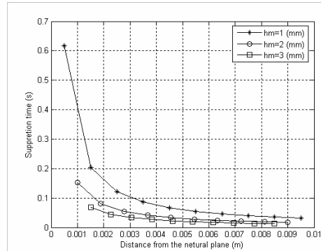
شکل (۱۲) منحنیهای زمان نشست بر حسب فاصله مختلف لایه‌های مگنتواستریتکیو از سطح میانی برای پوسته FGM فولاد- زیر کونیا
