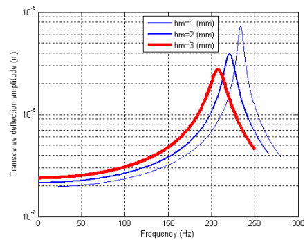
شکل (۱۰) منحنیهای پاسخ فرکانسی پوسته FGM فولاد- زیر کونیا برای مقادیر مختلف ضخامت لایه‌های مگنتواستریتکیو
