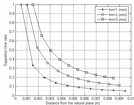
شکل (۱۴) منحنیهای نسبت زمان نشست بر حسب فاصله مختلف لایه‌های مگنتواستریتکیو از سطح میانی برای پوسته FGM فولاد- زیر کونیا
