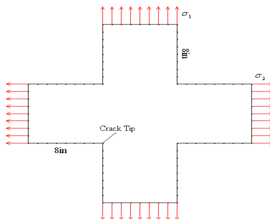
شکل (۸) صفحه صلیبی ترکدار
