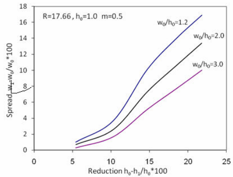
شکل (۶) تأثیر نسبت \frac{w_0}{h_0} روی تعریض در نورد تخت با فاکتور
