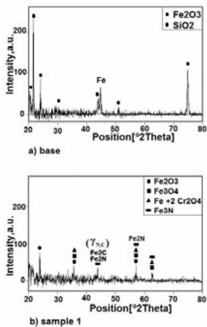
شکل ۲- طیف‌های XRD، a: نمونه‌ی بدون پوشش، b: نمونه‌ی نیتروکربور شده.
