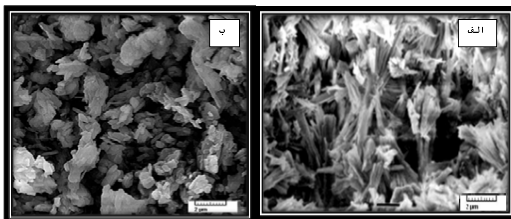
شکل ۷- تصویر SEM از الف) گچ مربوط به قالب کلسینه شده ب) گچ مربوط به قالبی که بخوبی خشک شده و کلسینه نشده
