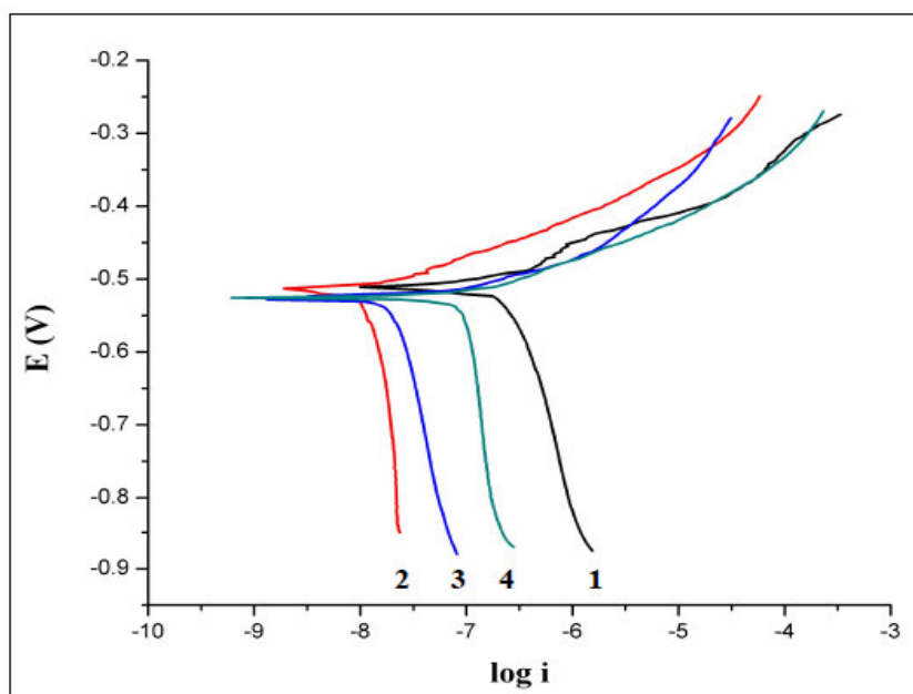
شکل 7- نمودار آزمون برون یابی تافل نمونه های 1 تا 4 مربوط به الکترولیت بهینه (الکترولیت (ب)).
