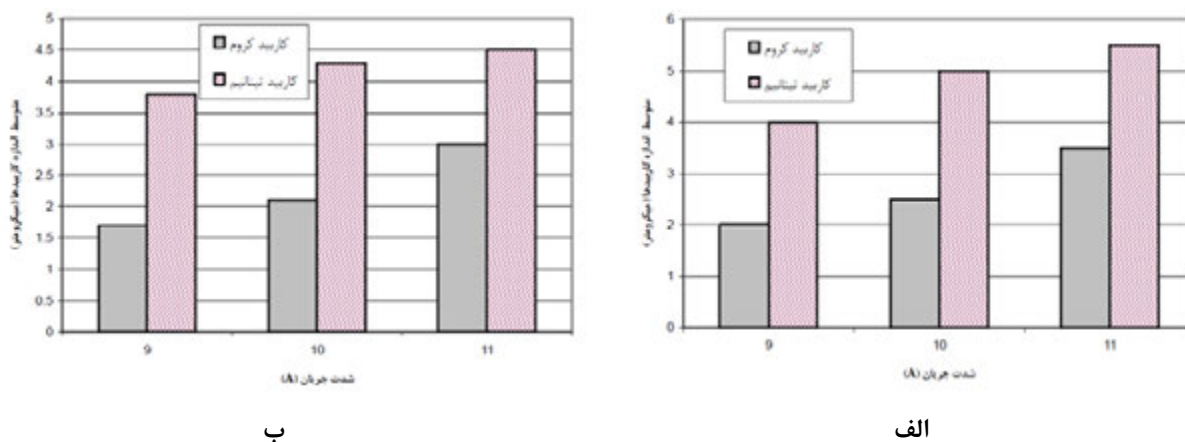
شکل 4- ارتباط بین اندازه میانگین کاربیدهای \text{Cr}_{23}\text{C}_6 و \text{TiC} بر حسب شدت جریان جوشکاری برای نمونه‌های گوناگون.
