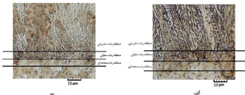
شکل 2- ریزساختار میکروسکوپی مرز ذوب نمونه جوشکاری شده با شدت جریان 9 آمپر.
