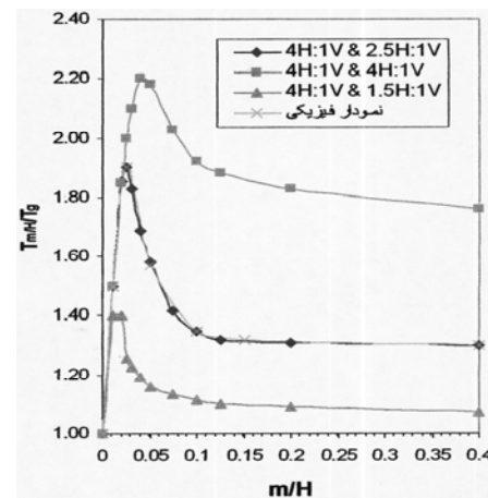
شکل ۱. نمودار نشان دهنده ی تغییرات m/H به T_{mH}/T_g بدست آمده از شبیه BREACH در پایین دست.
