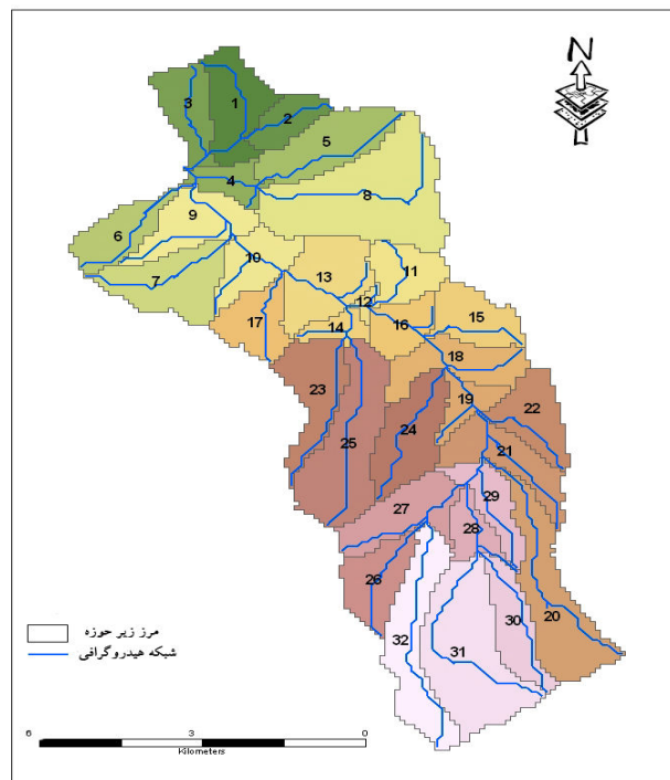
شکل ۴- شبکه‌ی آبنگاری و ۳۲ زیرحوضه‌ی مورد مطالعه‌ی حوضه‌ی آبخیز کسبلیان.
