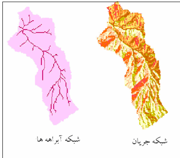
شکل ۳- ترسیم شبکه‌ی جریان و شبکه‌ی آبراهه‌های حوضه‌ی آبخیز کسبلیان با استفاده از برنامه‌ی HEC-Geo HMS.
