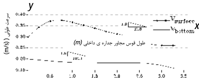
شکل 10. سرعت طولی مجاور جداره ی داخلی در قوس 4.
