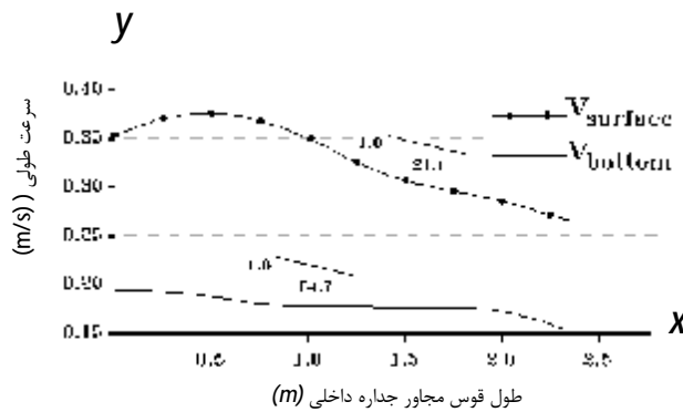
شکل 12. سرعت طولی مجاور جداره ی داخلی در قوس 3.
