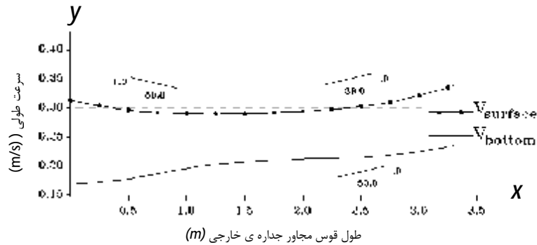
شکل 11. سرعت طولی مجاور جداره ی خارجی در قوس 3.
