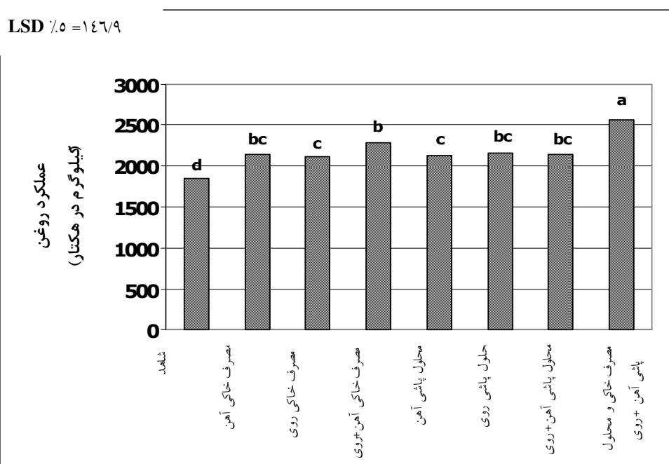
شکل ۵- اثر عناصر کم مصرف آهن و روی و روش مصرف آنها بر عملکرد روغن آفتابگردان
