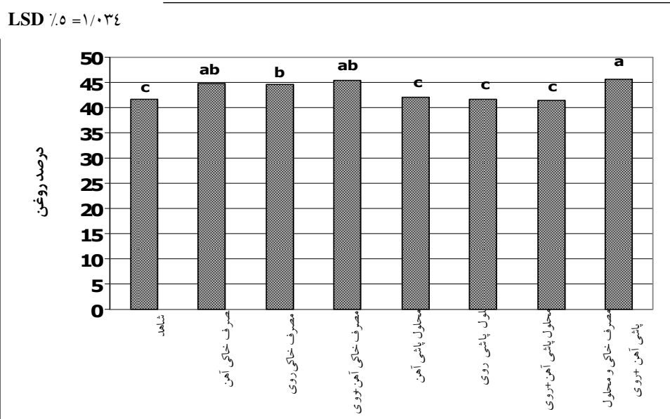
شکل ۴- اثر عناصر کم مصرف آهن و روی و روش مصرف آنها بر درصد روغن آفتابگردان
