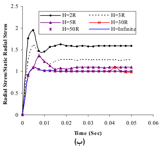
شکل ۵: (الف) تغییر مکان محیطی بدون بعد گره ۳۸ در طول زمان (ب) تنش محیطی بدون بعد گره ۳۸ در طول زمان.
