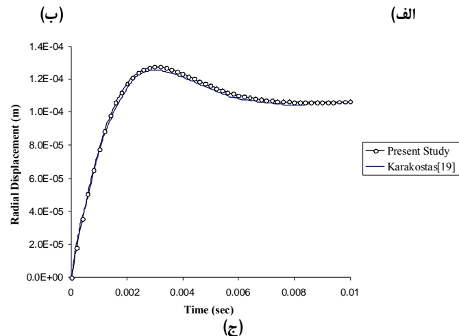
شکل ۱: تونل دایره ای تحت اثر انفجار ناگهانی: (الف) هندسه (ب) المان بندی (ج) تغییر مکان شعاعی.
