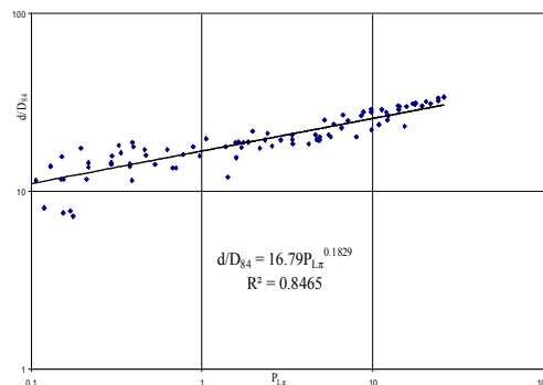
شکل ۶: رابطه بین P_{L\pi} و \frac{d}{D_e} برای ایستگاه هیدرومتری سیرا - کرج.
