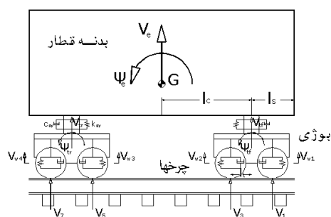
نمای طولی
