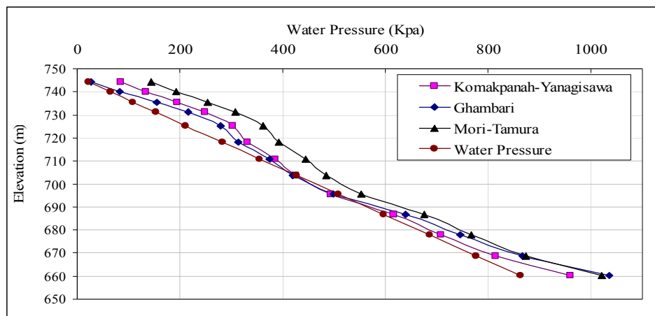
شکل ۱۳: مقایسه فشار آب ایجادکننده ترک حاصل از روابط مختلف با فشار آب در المان‌های بالادست هسته در زمان اولین آبیگری.
