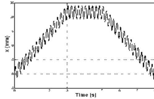
شکل ۶: نمودار تابع تحریک دوزنقه ای.
