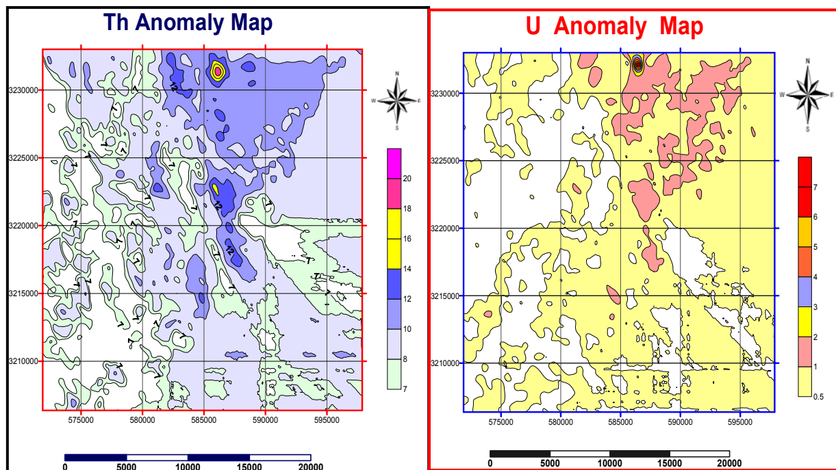
شکل ۵: نقشه های تفکیک آنومالی عناصر اورانیوم و توریم با واحد معادل گرم بر تن (ppm) در منطقه ده بگری
