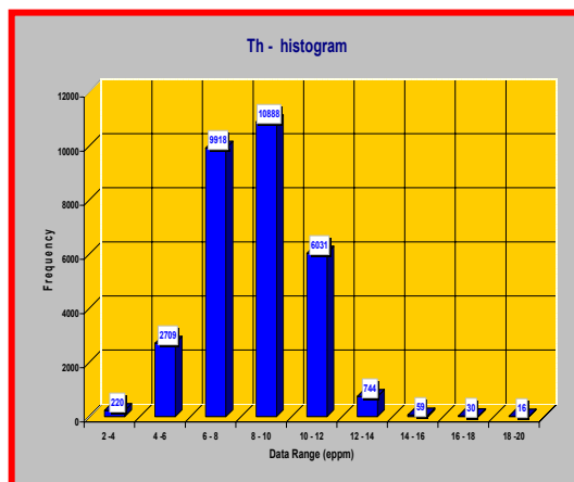
شکل ۳: نمودار هیستوگرام توزیع فراوانی داده‌های رادیومتری عنصر توریم (Th) منطقه ده بکری
