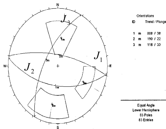
شکل ۶: تصویر استریوگرام دسته درزه های کیلومتر ۵۰/۷ تا کیلومتر ۵۰/۷۶ آزادراه
