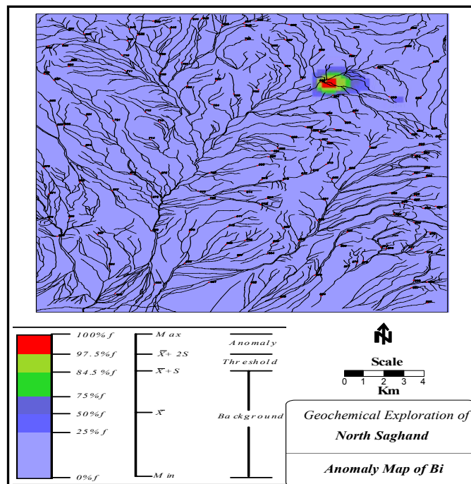
شکل ۵: نقشه ژئوشیمیایی آنومالی Bi در برگه ۱:۵۰۰۰۰ شمال ساغند (به روش حدآستانه‌ای)
