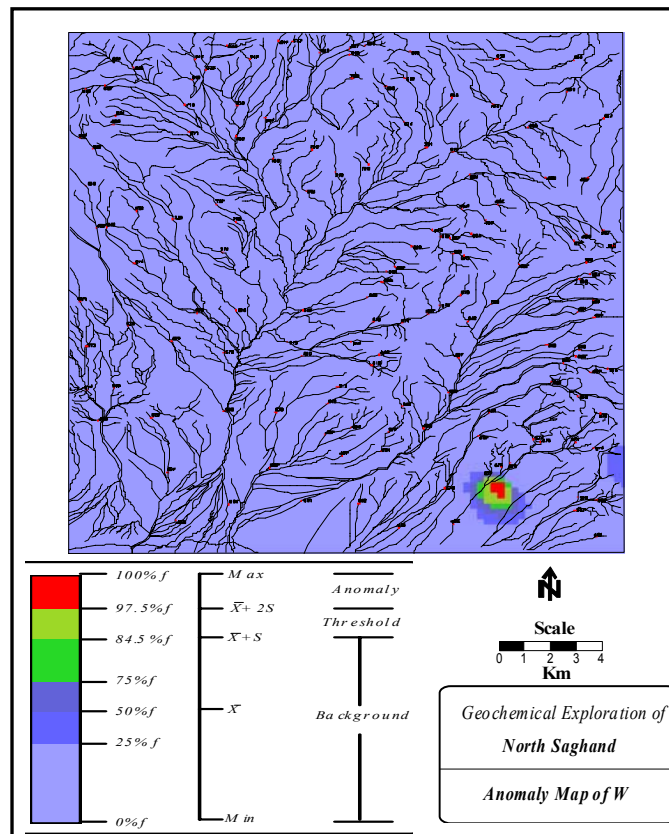
شکل ۴: نقشه ژئوشیمیایی آنومالی W در برگه ۱:۵۰۰۰۰ شمال ساغند (به روش حدآستانه‌ای)
