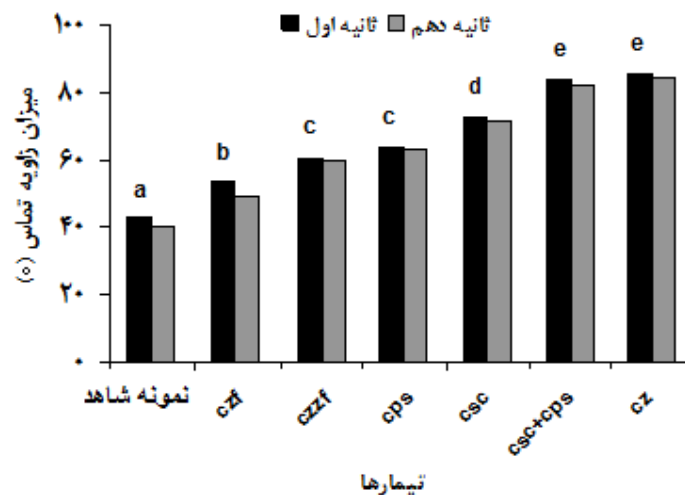
شکل ۵- میزان زاویه تماس اندازه گیری شده بر روی نمونه شاهد و نمونه های پوشش داده شده
