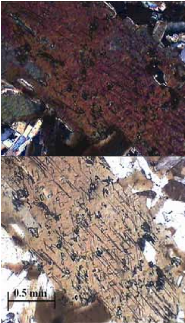
تصویر ۱۴- سوزن‌های روتیل در بیوتیت‌های گرانیت بن‌دونو و تشکیل فاسیس ساژنیتی (Sagenit texture). این بافت در اثر رشد بلورهای روتیل درون رخ‌ها با زاویه‌ی ۶۰ درجه ایجاد می‌شوند (نور طبیعی = PPL، نور پلاریزه = XPL)
