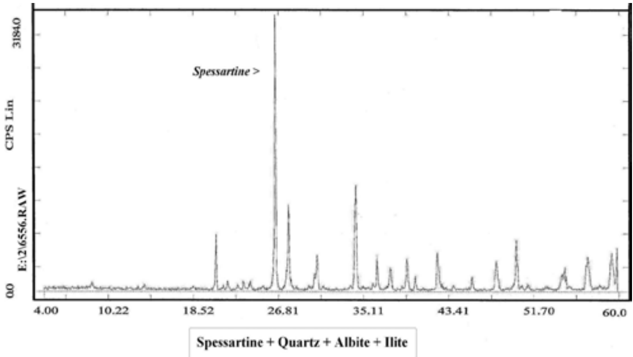
تصویر ۴- تجزیه‌ی کانی‌شناسی (XRD) که مشخص‌کننده‌ی نوع گارنت‌های بن‌دونو (Spessartine) است. فازهای فرعی گزارش شده شامل کوارتز، آلپیت و ایلپیت می‌باشند
