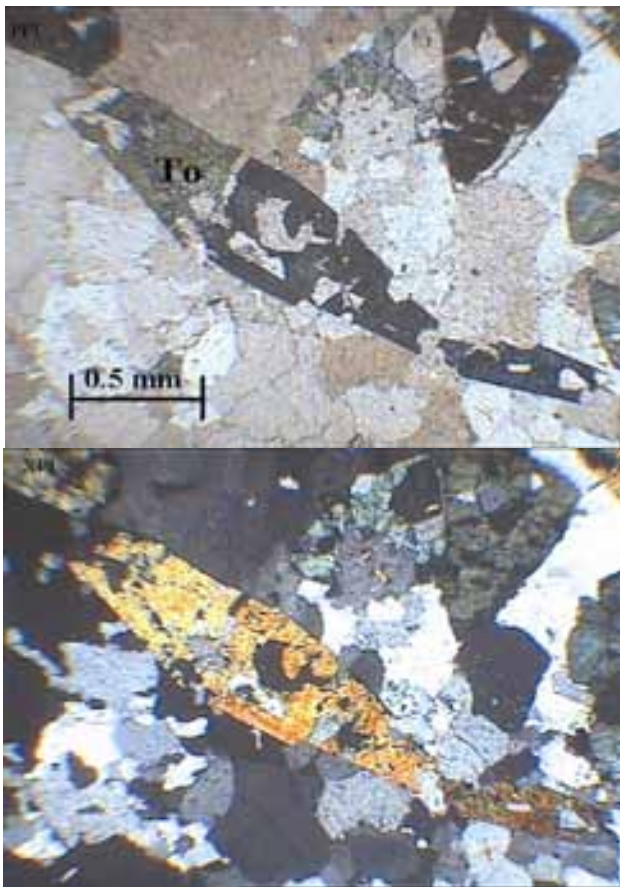
تصویر ۶- کانی تورمالین (Tourmaline) در آپلیت بن‌دونو. بلورهای تورمالین منطقه اغلب سوزنی شکل و اندازه‌ی آن‌ها بعضاً به چند سانتی‌متر می‌رسد. (نور طبیعی = PPL، نور پلاریزه = XPL)
