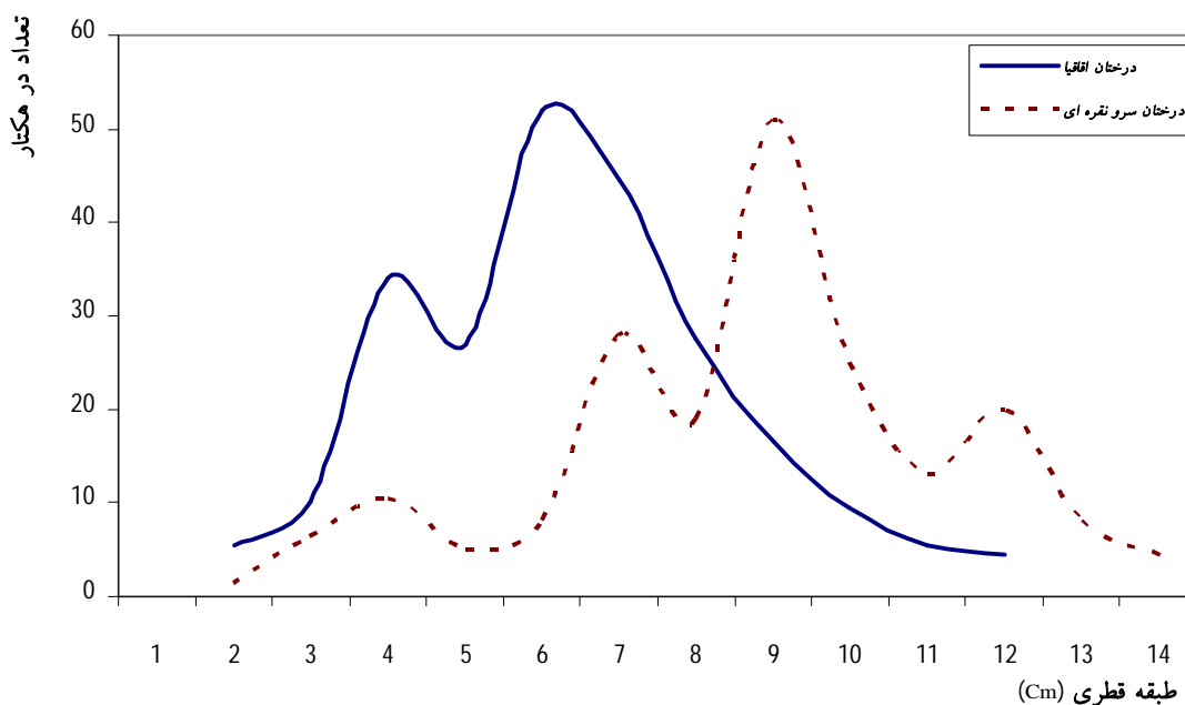
شکل 3- منحنی پراکنش تعداد در طبقات قطری درختان افاقیا و سرو نقره‌ای در منطقه مورد مطالعه
