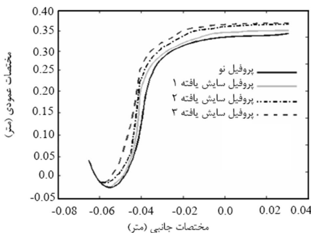
شکل 17 هندسه پروفیل‌های چرخ S1002 در چهار حالت نو، ساییش یافته 1، ساییش یافته 2 و ساییش یافته 3
