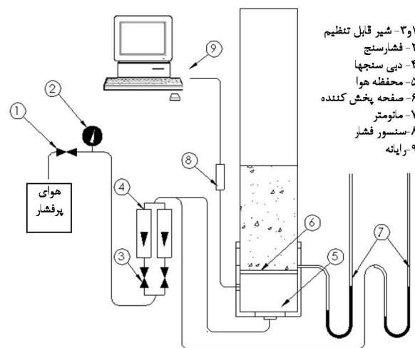
شکل 1 طرح‌واره‌ای از بستر مورد استفاده
