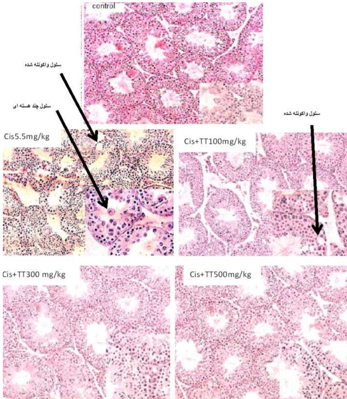
شکل ۲- مقایسه لوله‌های اسپرم‌ساز گروه‌های مختلف از لحاظ وجود سلول‌های چند هسته‌ای و واکنله شده (بزرگنمایی ۱۰۰×). هم-چنین بزرگنمایی ۴۰۰ این مقاطع در گوشه پائین و راست هر تصویر آورده شده است.
