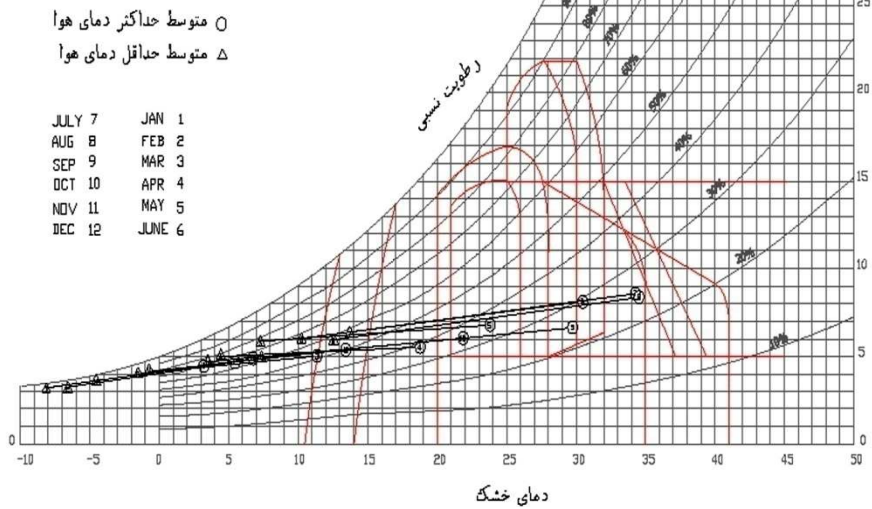
نمودار شماره ۲: بیوکلیماتی ساختمانی ایستگاه فرودگاه همدان منبع: داده‌های سی ساله آماری ایستگاه سینوپتیک فرودگاه همدان (۱۹۷۶ تا ۲۰۰۳)
