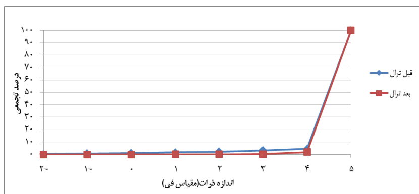
شکل ۲: نمودار تجمعی رسوبات در عمق ۶ متر در مقیاس Ø در منطقه بحرکان در سال ۱۳۸۹
