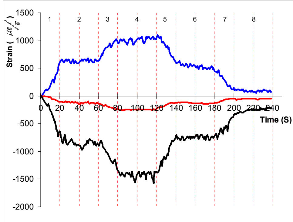
شکل ۳- کرنشهای رهاشده از سوراخکاری اولین نمونه متقارن متعامد [0_2 / 90_2]_S
