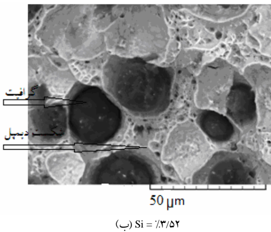
شکل (۶): تصویر تهیه شده توسط میکروسکوپ الکترونی روبشی از سطوح شکست نمونه‌های ضربه با مقادیر سیلیسیم متفاوت دمای 200^{\circ}\text{C} .
