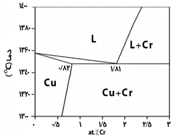
شکل (۱): دیاگرام فاز مس- کروم.
