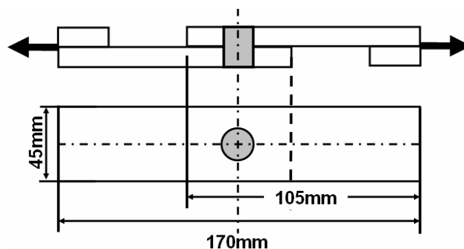
شکل (۱): ابعاد آزمایش کشش - برش.
