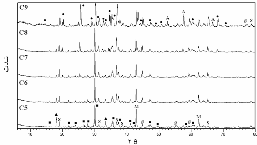
شکل (۳): نتایج آنالیز فازی سیمان‌های فرآوری شده با استفاده از دولومیت کلسینه شده پس از سینترینگ ■: CA, ●: CA 2 , ▲: C 12 A 7 , S: Spinel, M: MgO, A: Al 2 O 3
