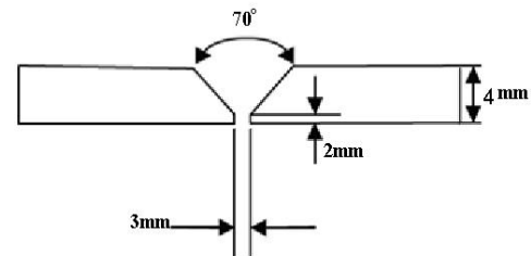
شکل (۱): طرح اتصال لوله ها.
