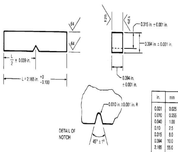
شکل (۳): جزییات نمونه برای آزمون ضربه طبق استاندارد AWS B4.0 [۸].
