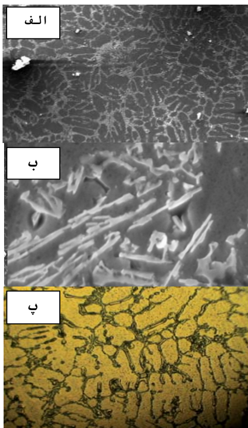
شکل (۲): ریزساختار نمونه‌های ریخته‌گری شده در دمای 75^{\circ}\text{C} با اندازه ذرات 300\ \mu\text{m} : (الف) تصویر SEM با بزرگنمایی 200\times ، (ب) تصویر SEM با بزرگنمایی 2000\times و (پ) تصویر میکروسکوپ نوری با بزرگنمایی 400\times
