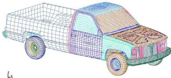
شکل (۱): مدل المان محدود خودروی مورد تحلیل
