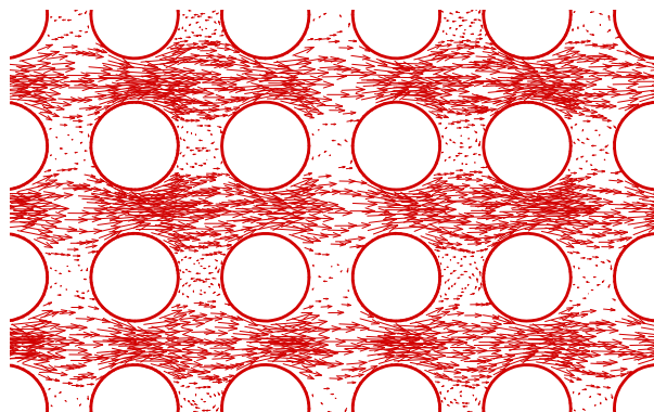
شکل(۶): بردارهای سرعت ( Re = 40000 )
