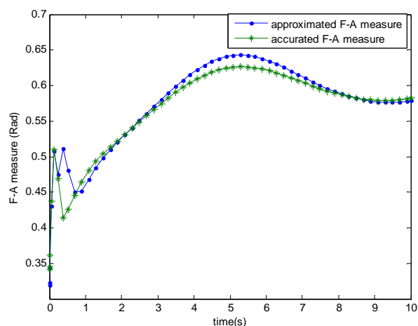
نمودار (۱۱): مقدار تخمینی و دقیق پایداری واقعی با توجه به کنترلر شکل (۱۳) در حالتی که چرخش اربابه غیربهینه ( \phi = -\pi/6 \cos(\pi/10) ) است
