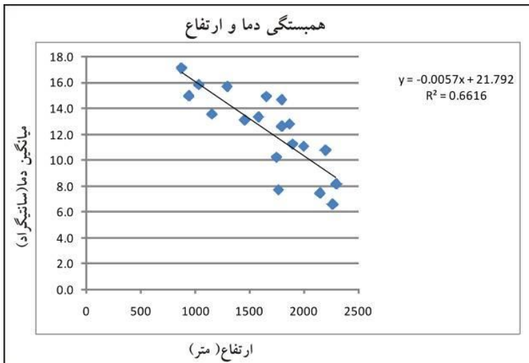
شکل 2 گرادیان دما در حوضه جاجرود با استفاده از داده‌های ایستگاه‌های موجود
