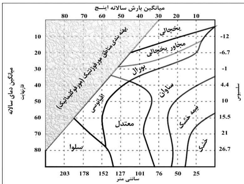
شکل 5 نمودار مناطق مورفوزنتیک پلتیر
