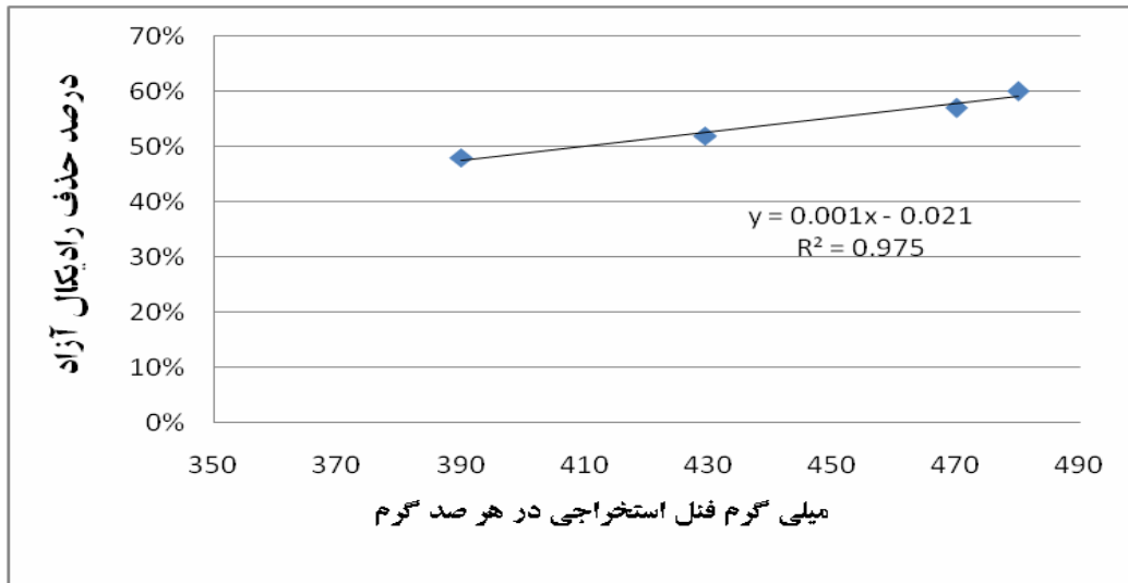
نمودار ۲- رابطه میان درصد کاهش رادیکال آزاد و میزان ترکیبات فنلی موجود در نمونه‌ها
